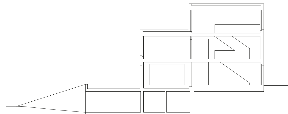
LÄNGSSCHNITT__LONGITUDINAL SECTION
